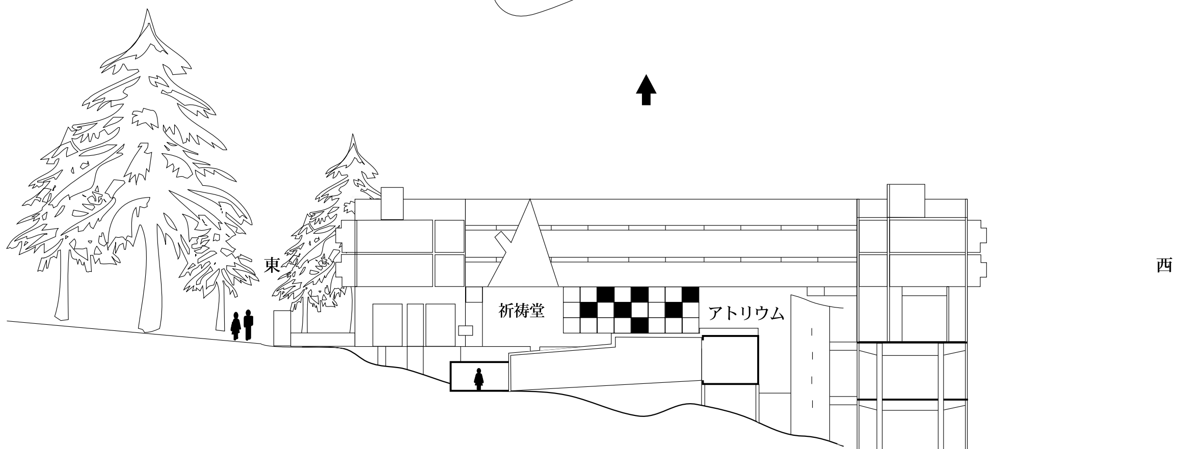
北側立面図
